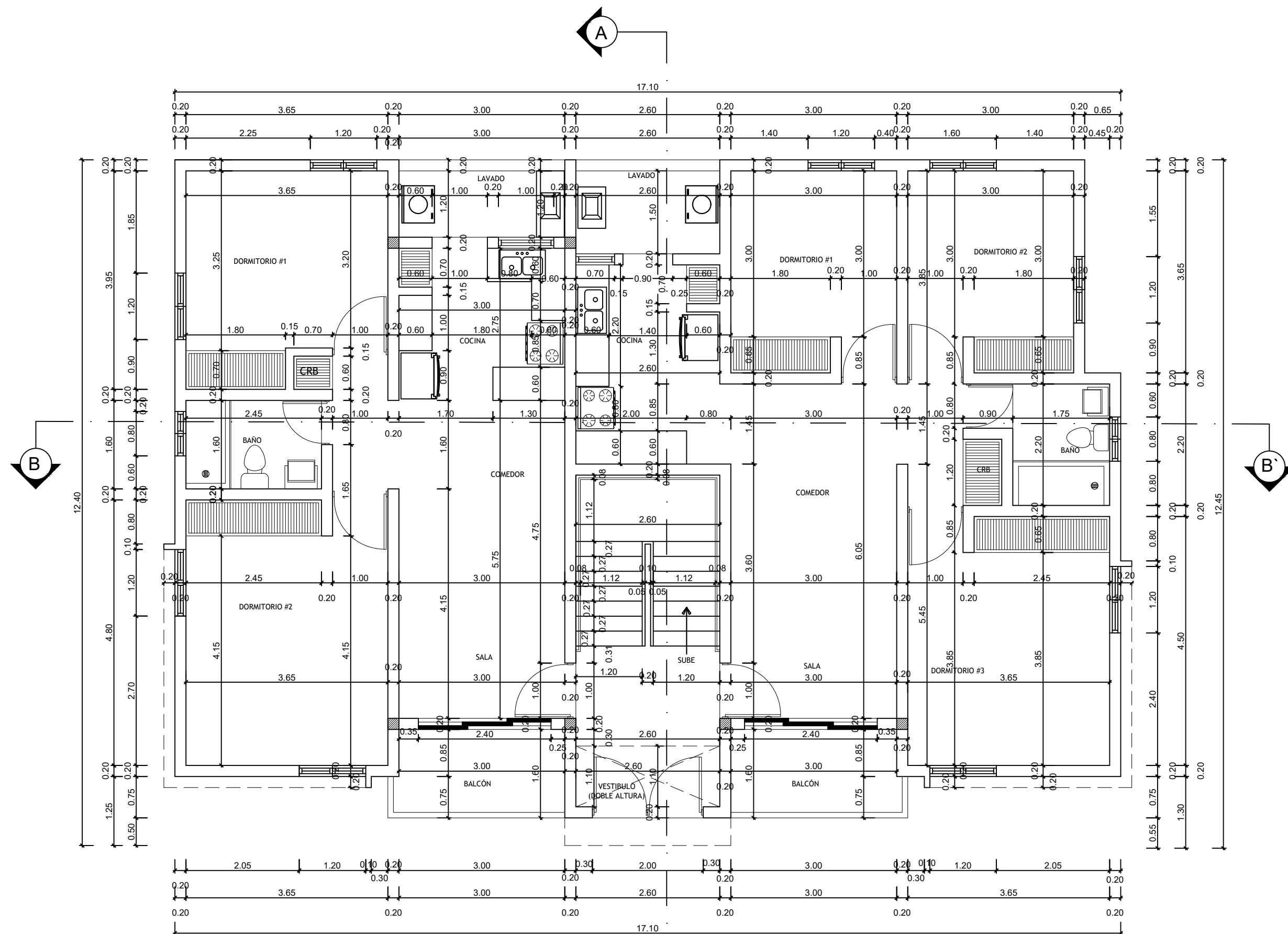
PLANTA DIMENSIONADA 1ER. NIVEL, BLOQUE A ESCALA: 1:75
