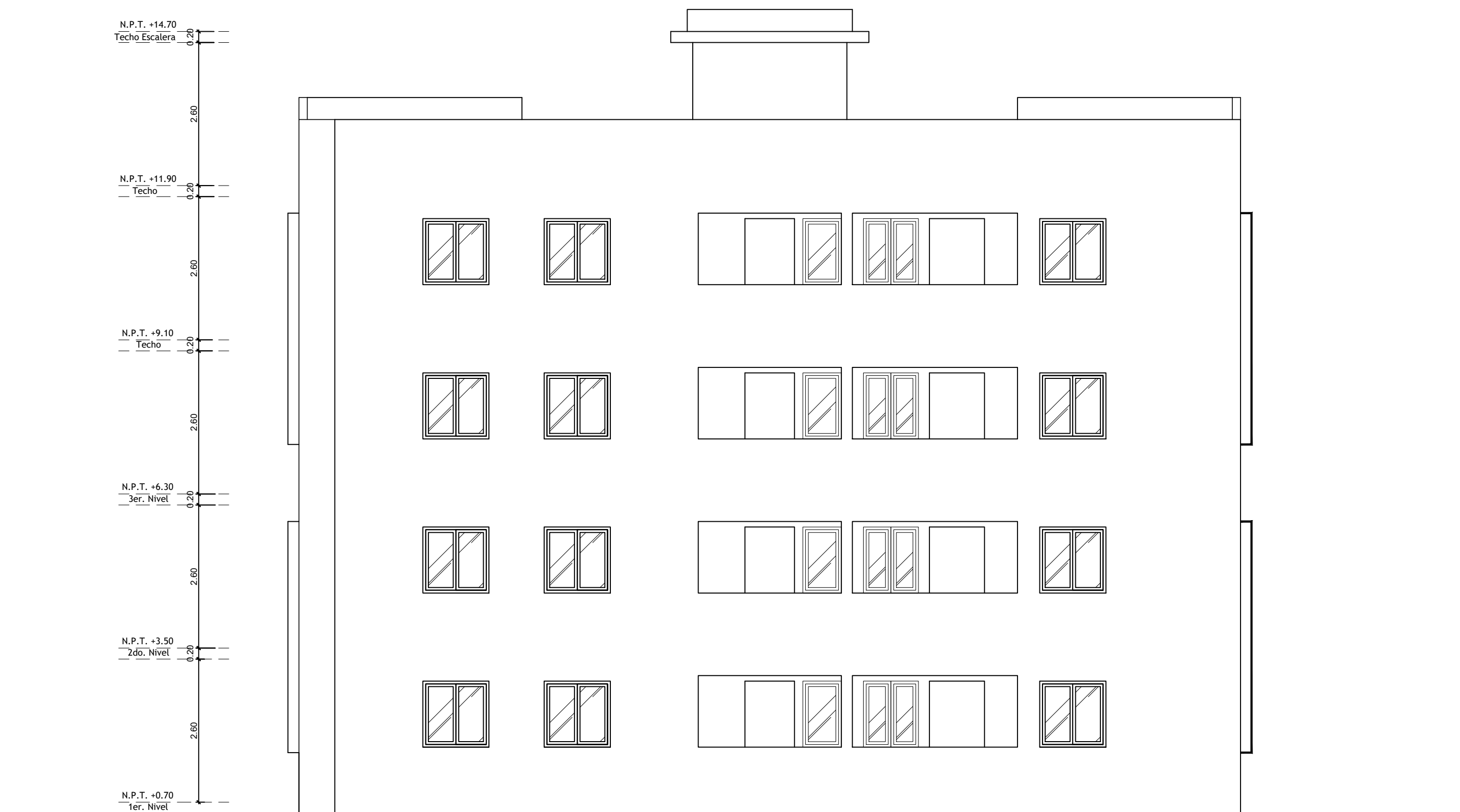
ELEVACION POSTERIOR, BLOQUE A ESCALA: 1:75
