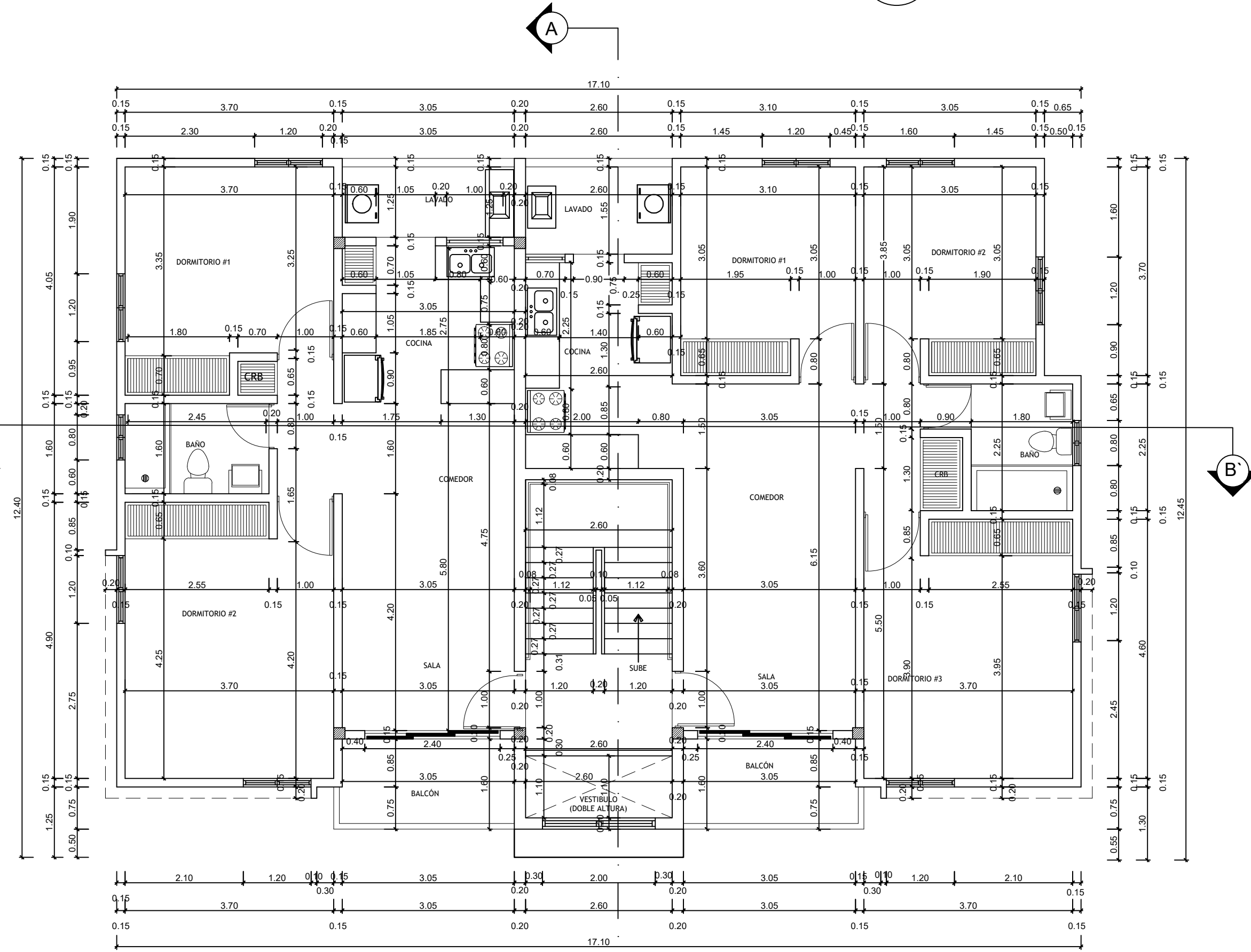
PLANTA DIMENSIONADA 2DO. NIVEL, BLOQUE A ESCALA: 1:75
