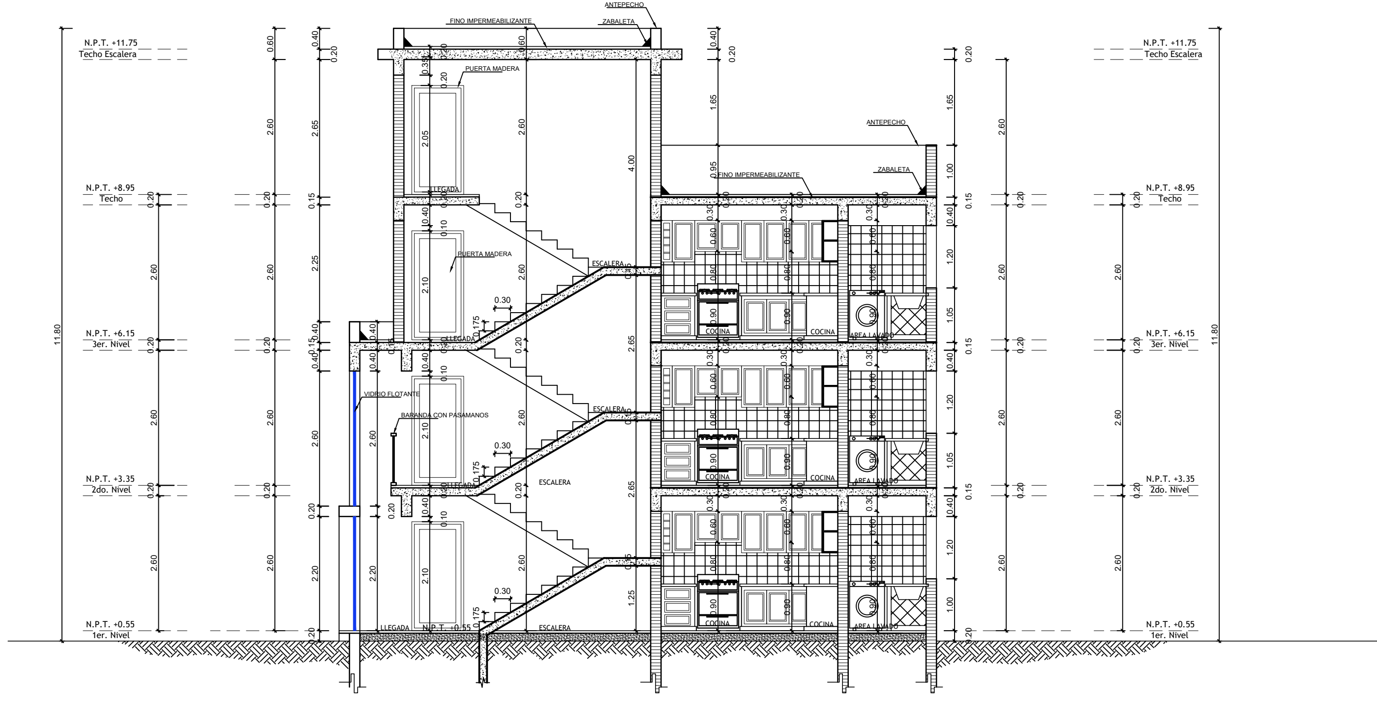
SECCION A-A', BLOQUE B ESCALA: 1:75
