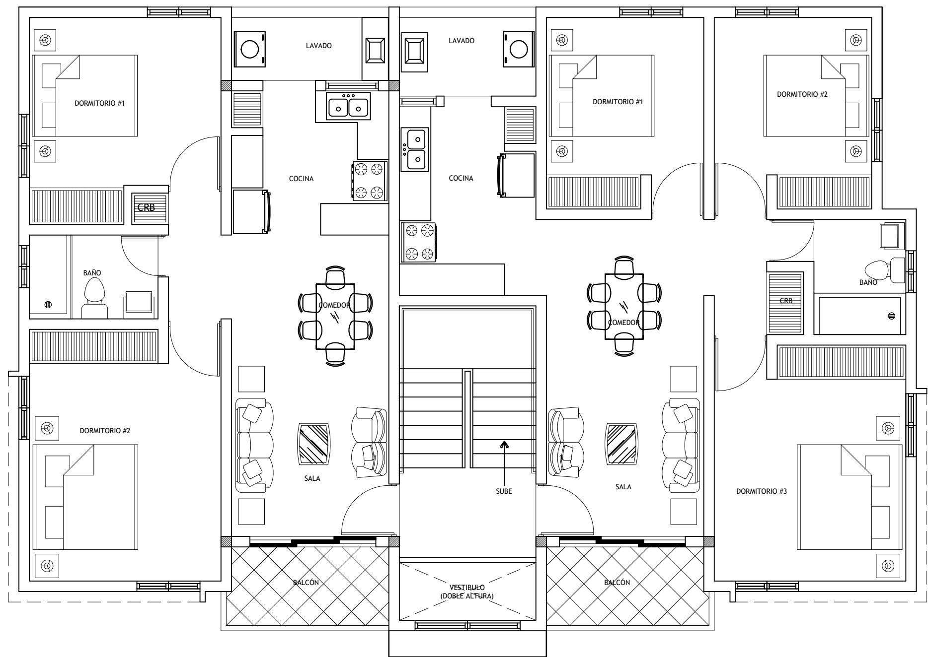
PLANTA ARQUITECTONICA 3ER. NIVEL, BLOQUE A ESCALA: 1:75
