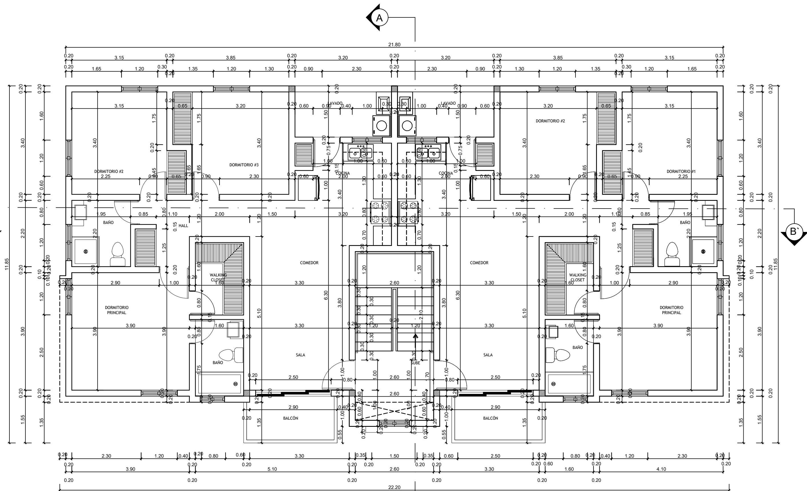
PLANTA DIMENSIONADA 2DO. NIVEL, BLOQUE B ESCALA: 1:75
