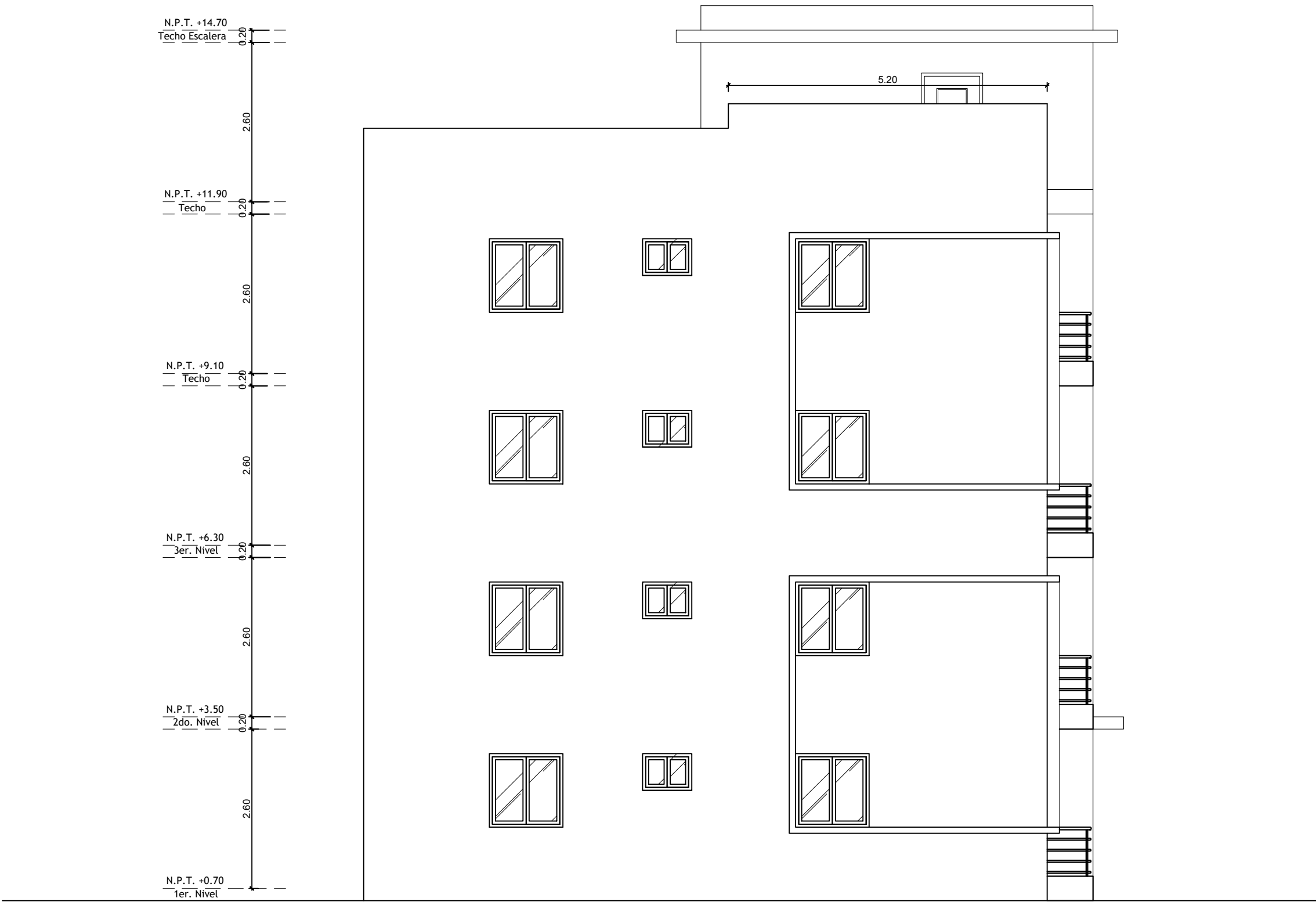
ELEVACION LATERAL IZQUIERDO, BLOQUE A ESCALA: 1:75
