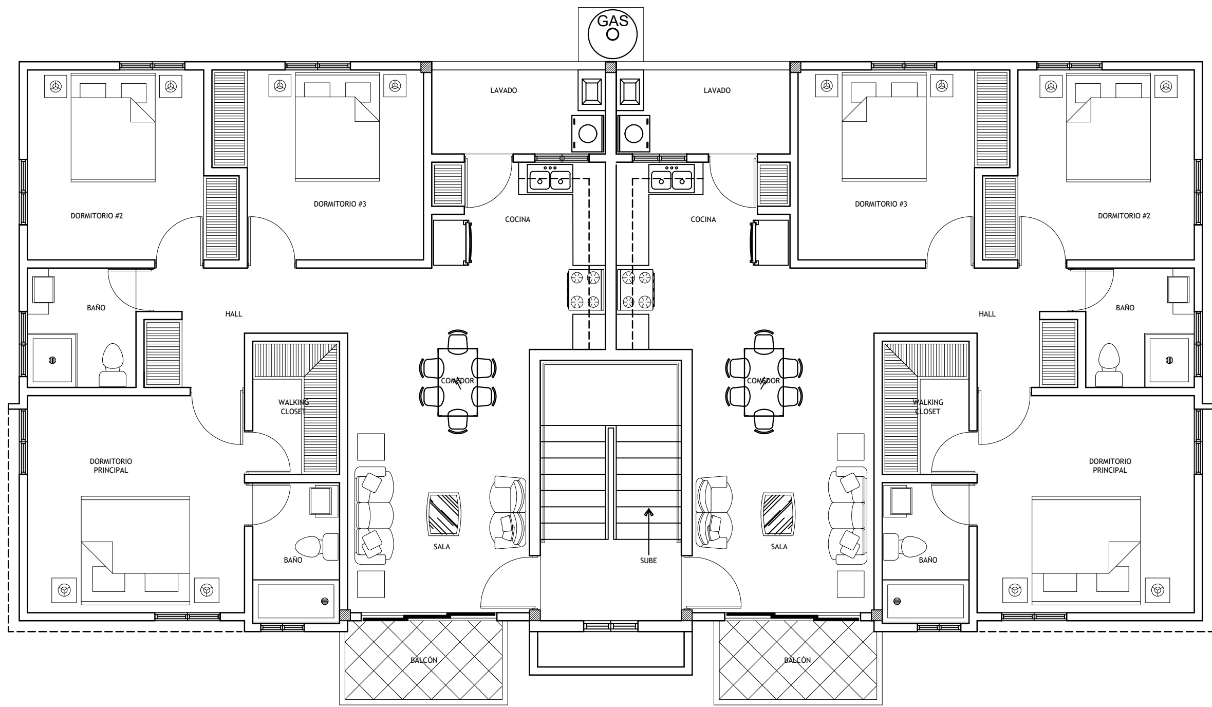
PLANTA ARQUITECTONICA 3ER. NIVEL, BLOQUE B ESCALA: 1:75
