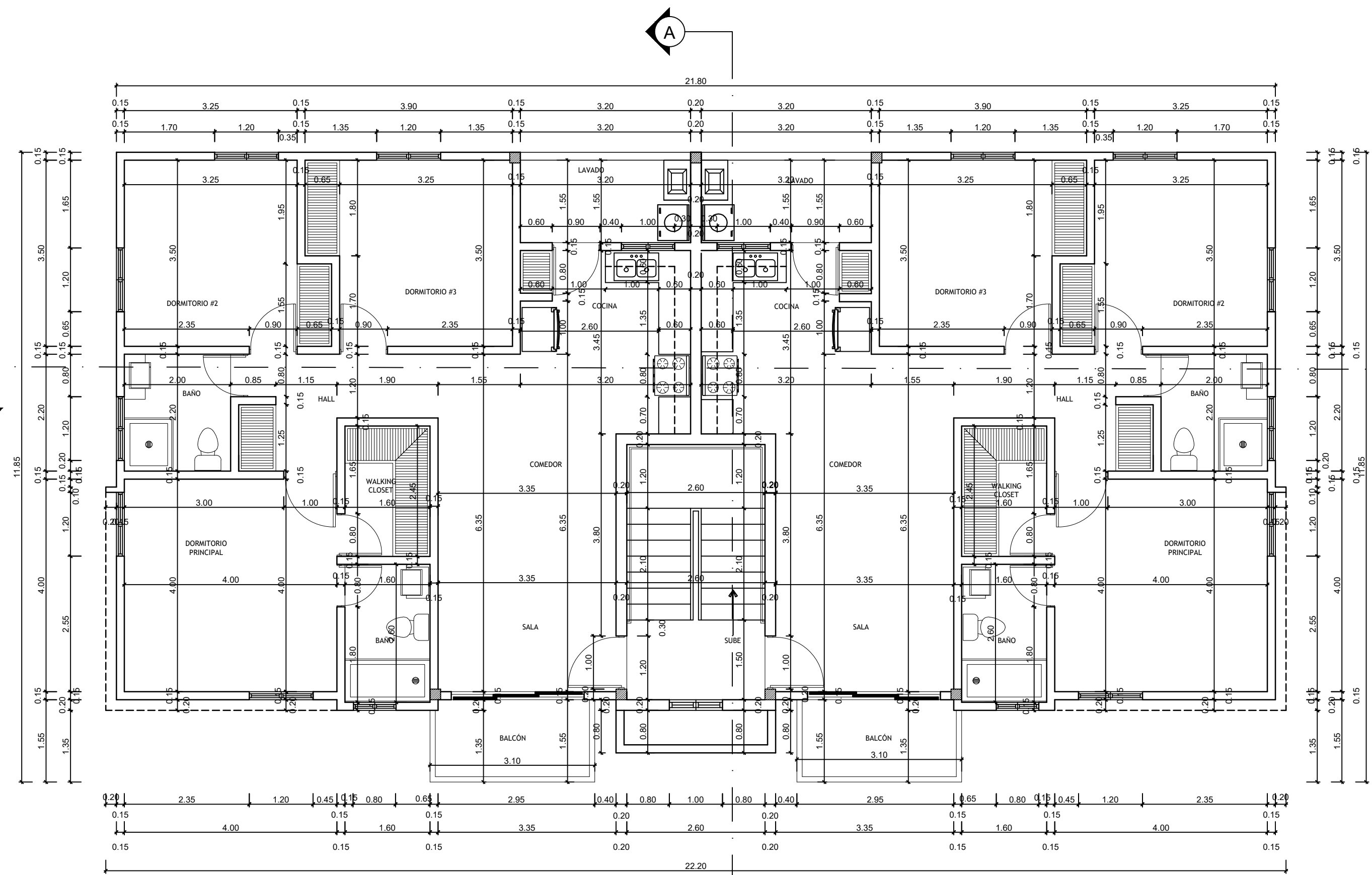
PLANTA DIMENSIONADA 3ER. NIVEL, BLOQUE B ESCALA: 1:75
