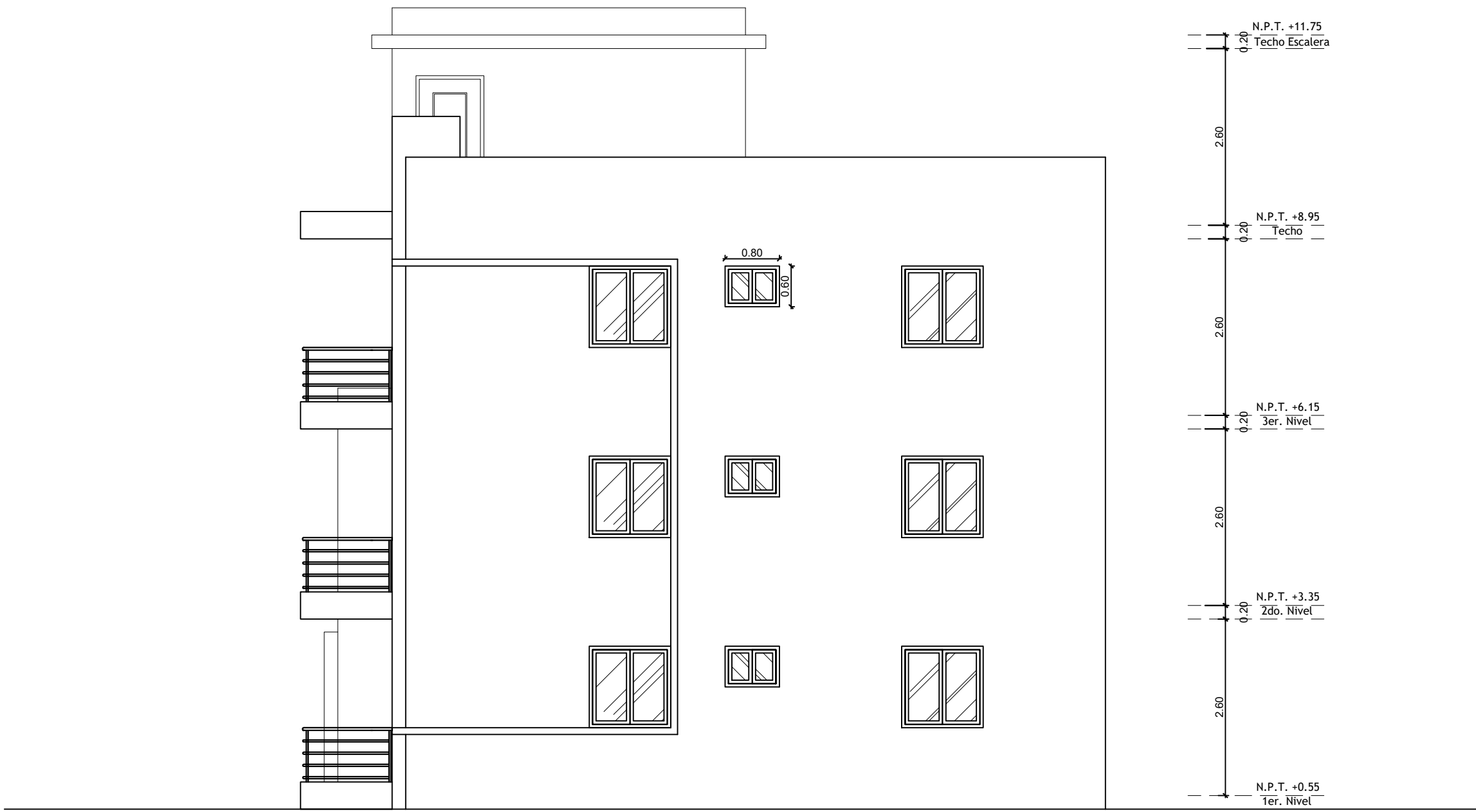
ELEVACION LATERAL DERECHO, BLOQUE B ESCALA: 1:75
