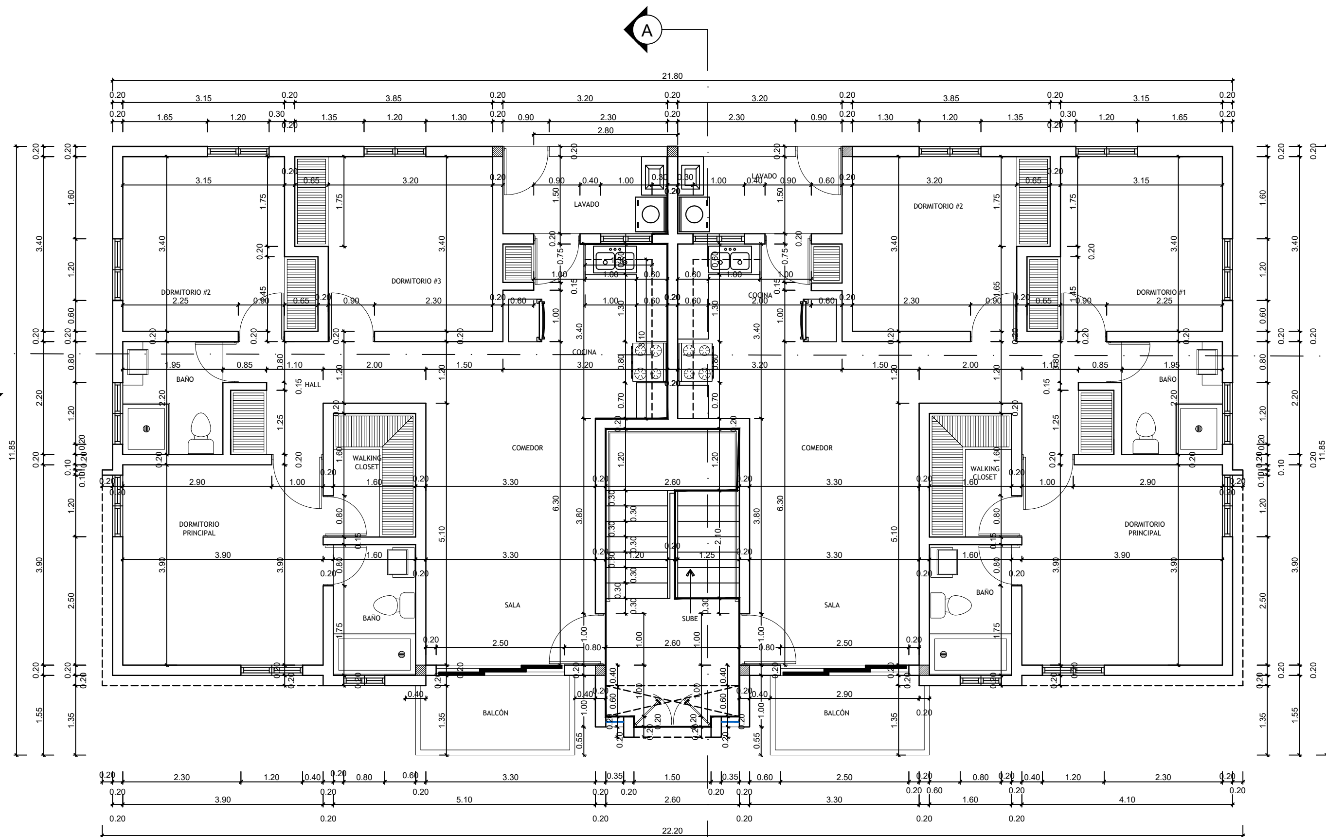
PLANTA DIMENSIONADA 1ER. NIVEL, BLOQUE B ESCALA: 1:75
