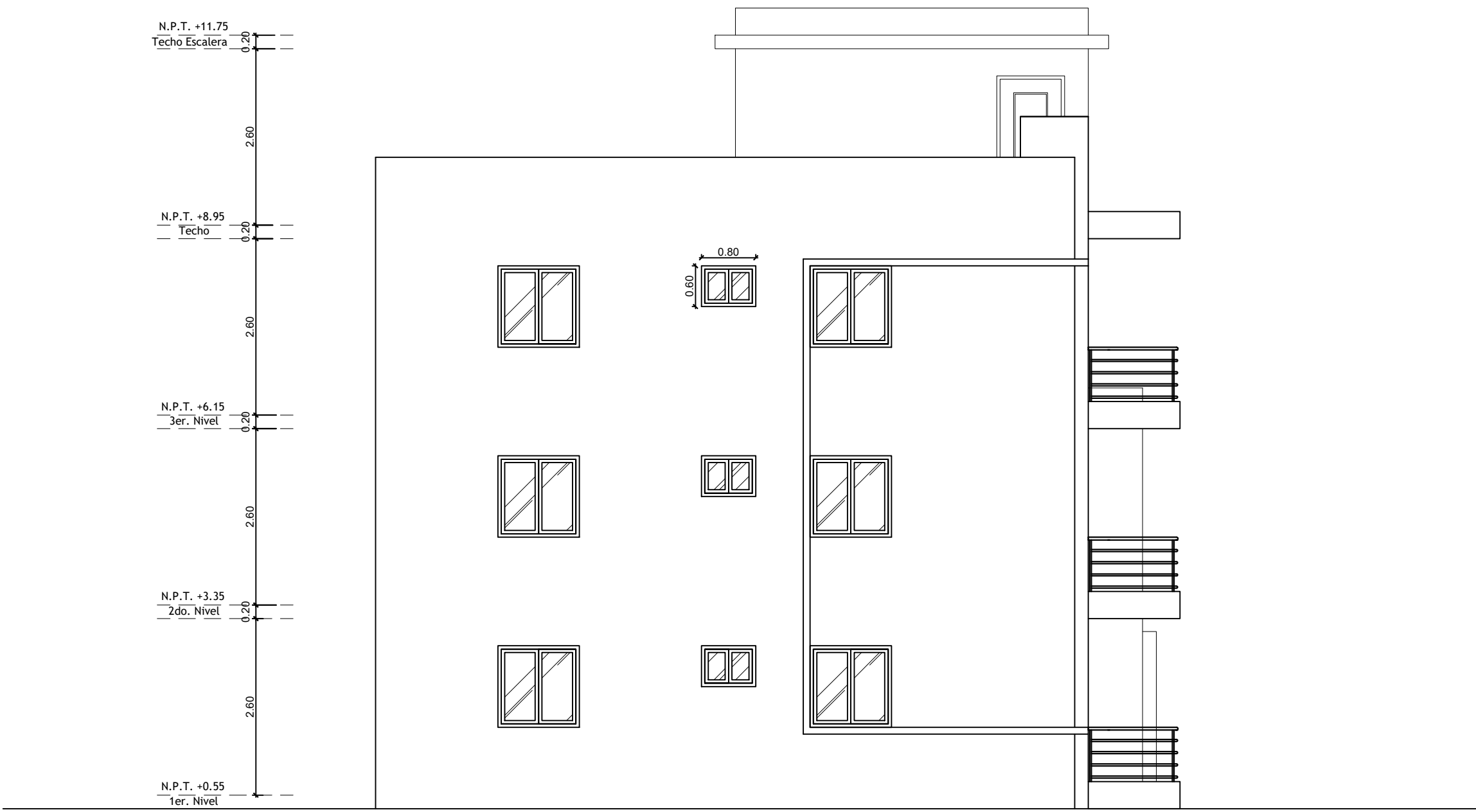
ELEVACION LATERAL IZQUIERDO, BLOQUE B ESCALA: 1:75
