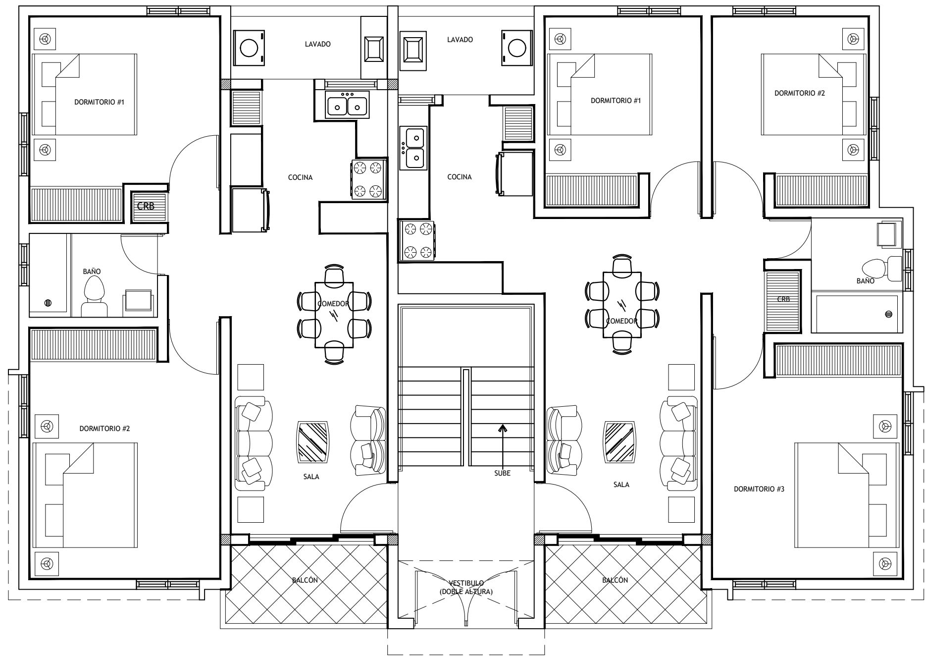
PLANTA ARQUITECTONICA 1ER. NIVEL, BLOQUE A ESCALA: 1:75
