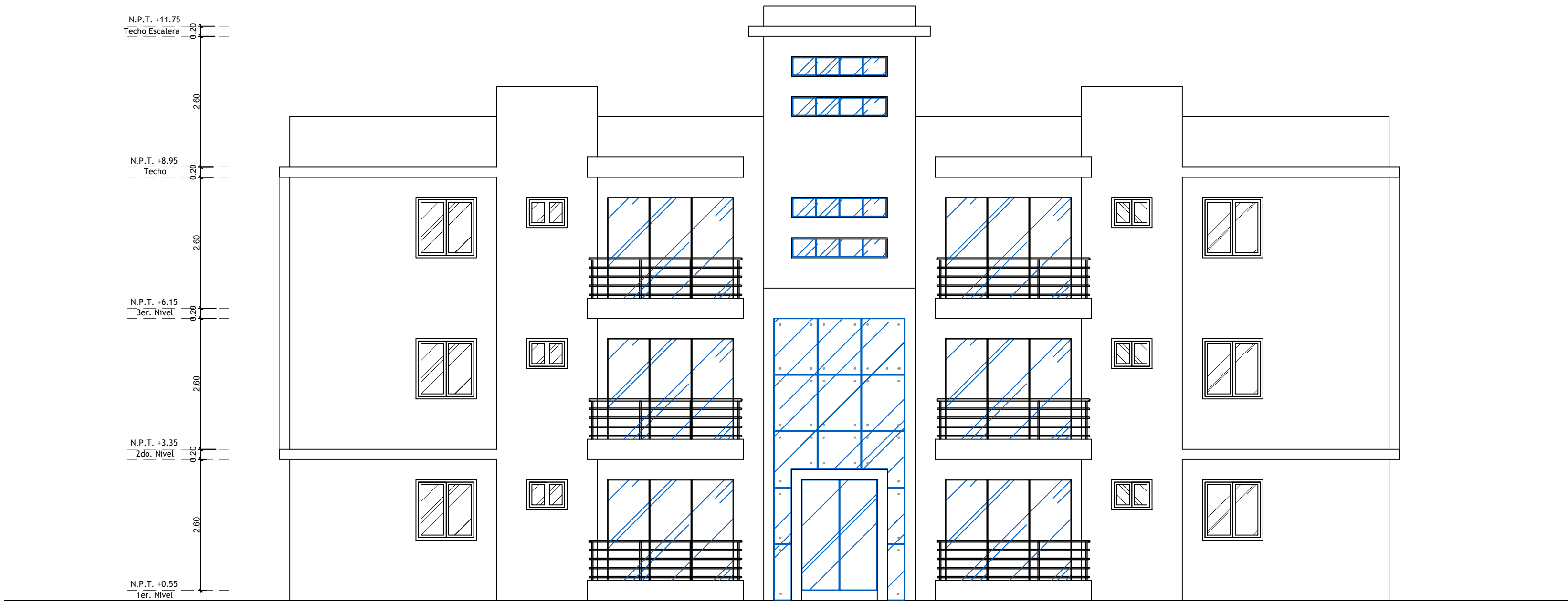
ELEVACION FRONTAL, BLOQUE B ESCALA: 1:75
