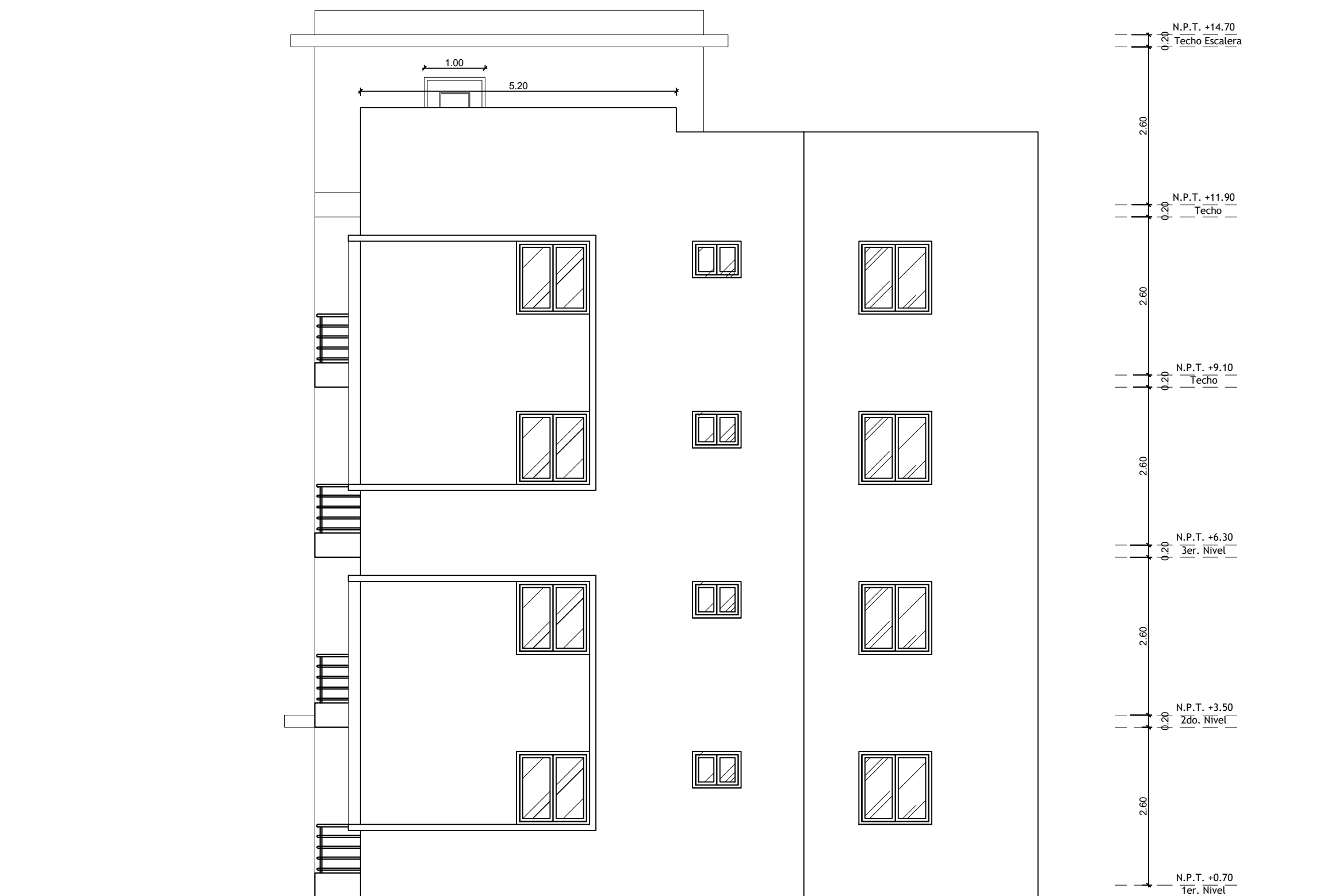
ELEVACION LATERAL DERECHO, BLOQUE A ESCALA: 1:75
