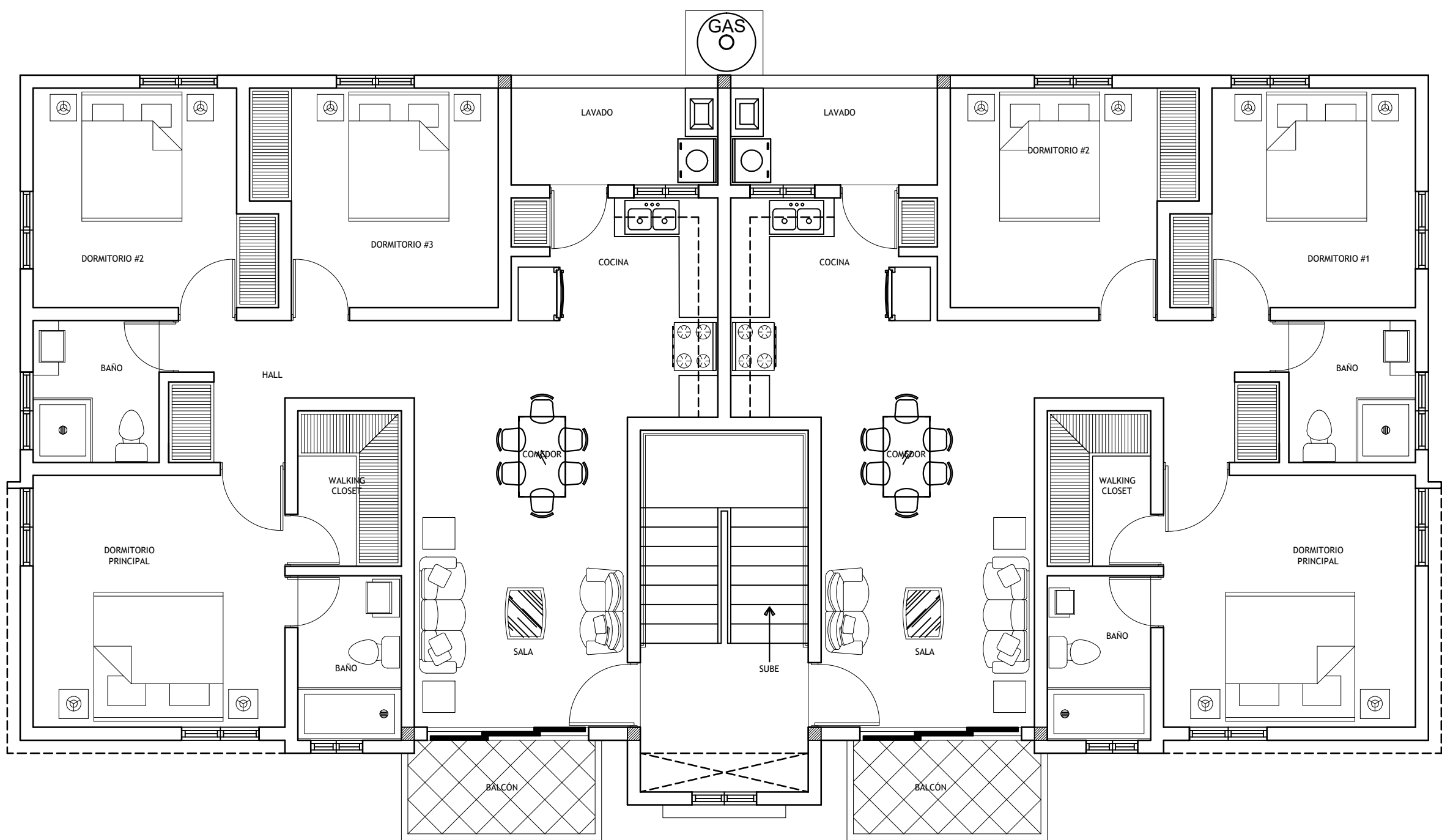
PLANTA ARQUITECTONICA 2DO. NIVEL, BLOQUE B ESCALA: 1:75
