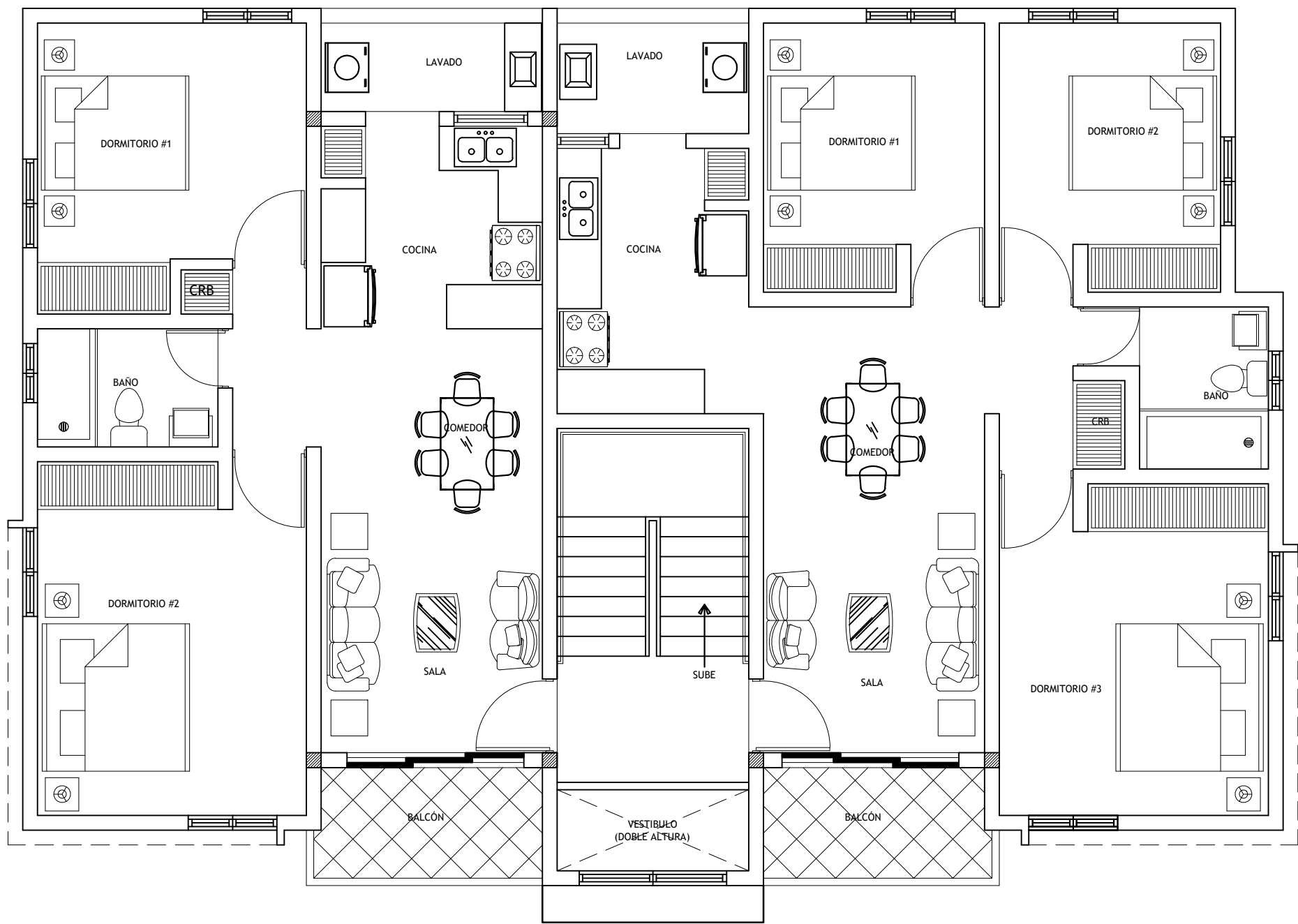
PLANTA ARQUITECTONICA 2DO. NIVEL, BLOQUE A ESCALA: 1:75
