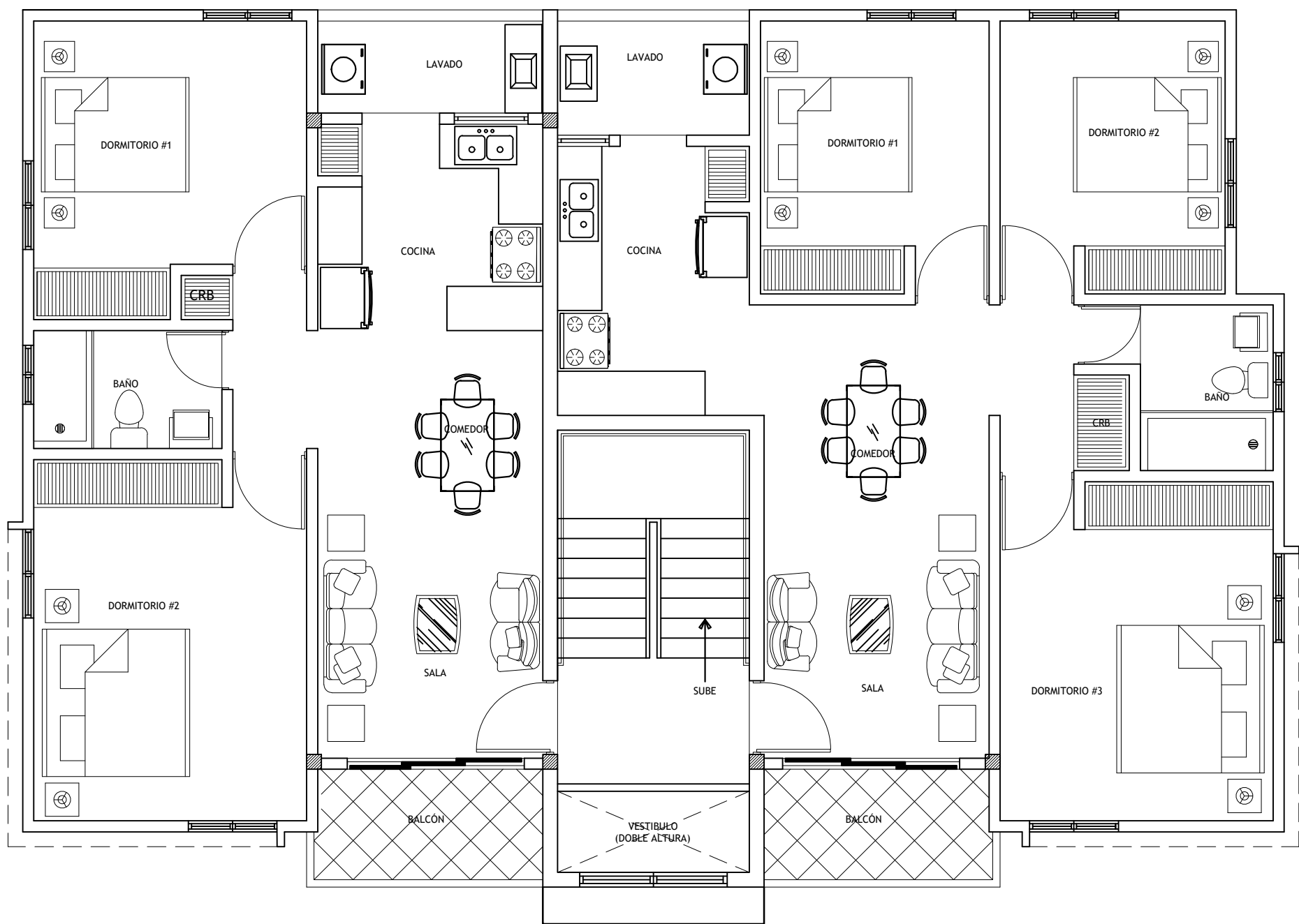
PLANTA ARQUITECTONICA 4TO. NIVEL, BLOQUE A ESCALA: 1:75
